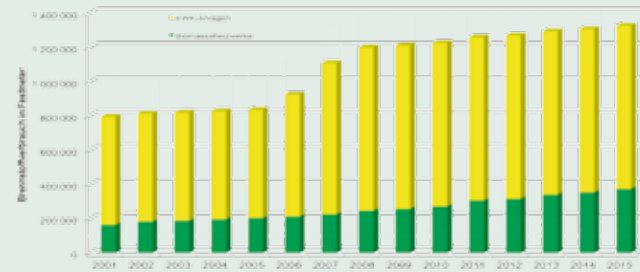
Brennstoffbedarf für Biomasseheizwerke und KWK-Anlagen auf Basis Holz in fm
